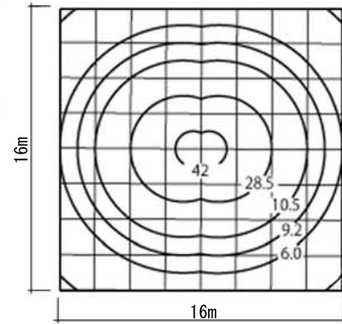
水平面照度分布図表 LED60W 2灯式
